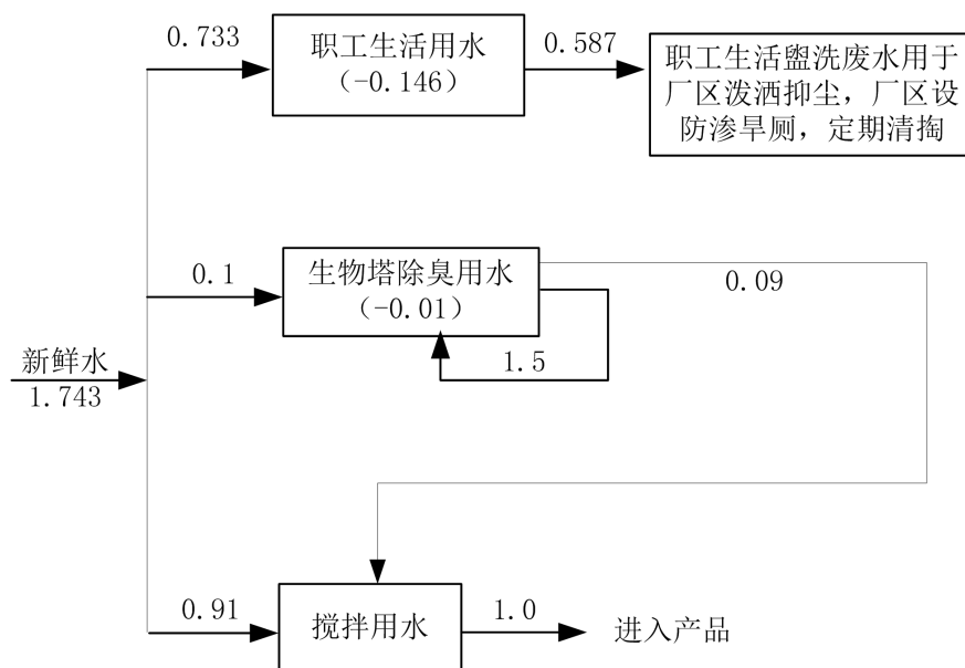
图 2-1 本项目给排水平衡图单位：m³/d
