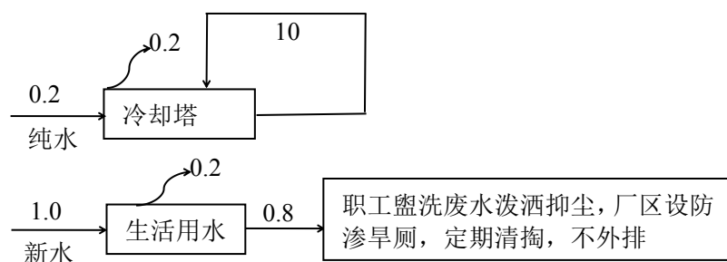
图 2-1 项目给排水平衡图 (单位： \text{m}^3/\text{d} )
