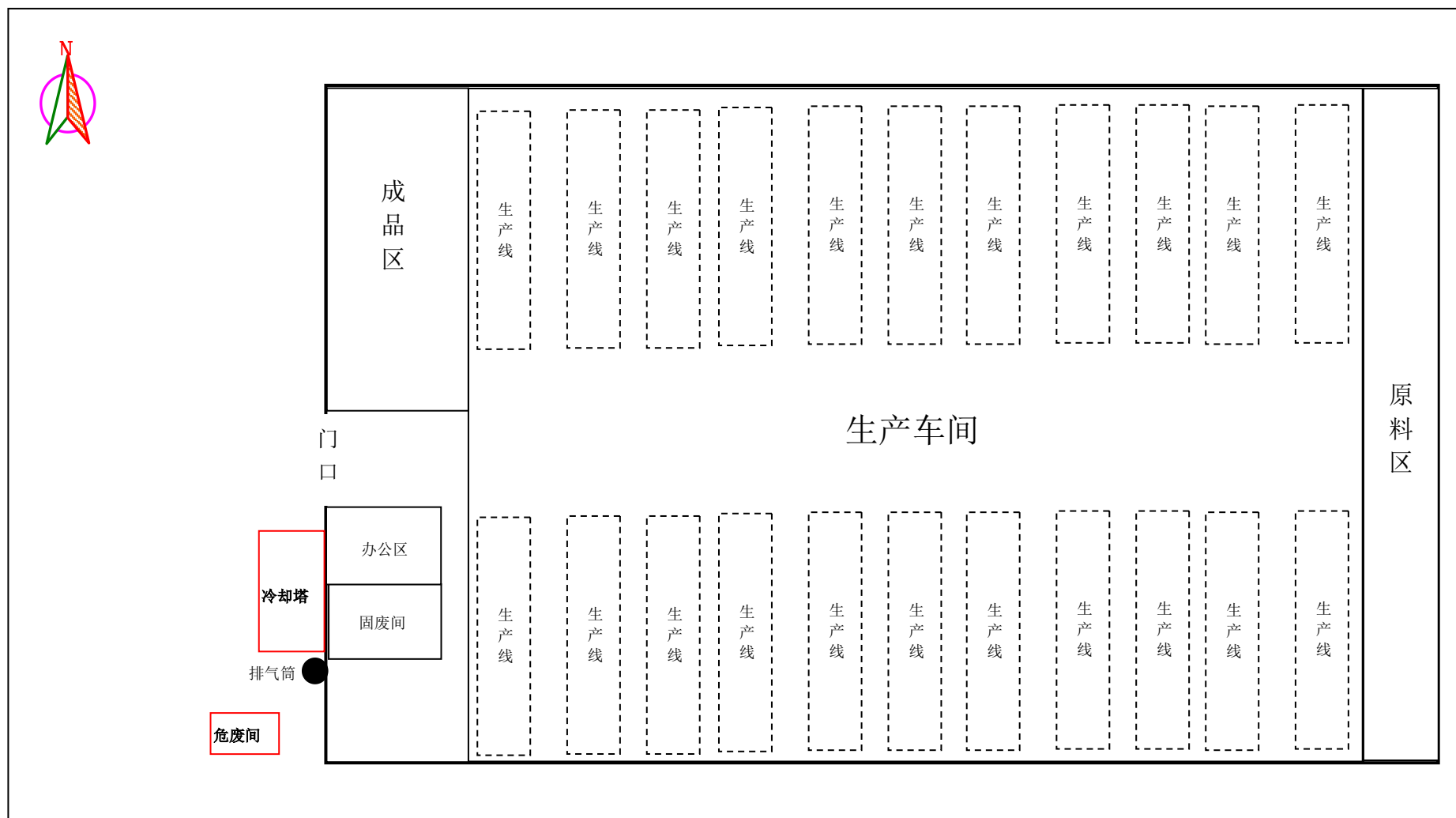
附图 4 项目平面布置图 比例 1:300
