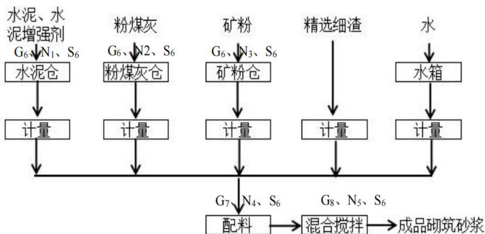
图 2-6 现有砌筑砂浆生产线产排污节点图
