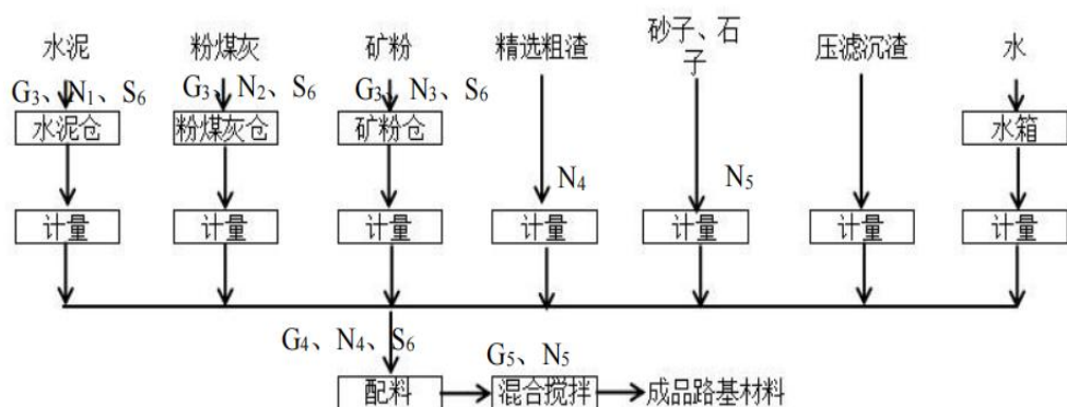
图 2-5 现有路基材料生产线产排污节点图
