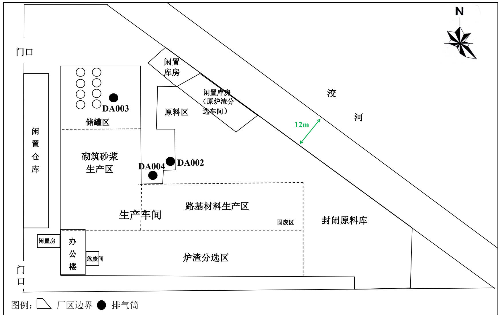
附图3 企业现有平面布置图 比例 1:900
