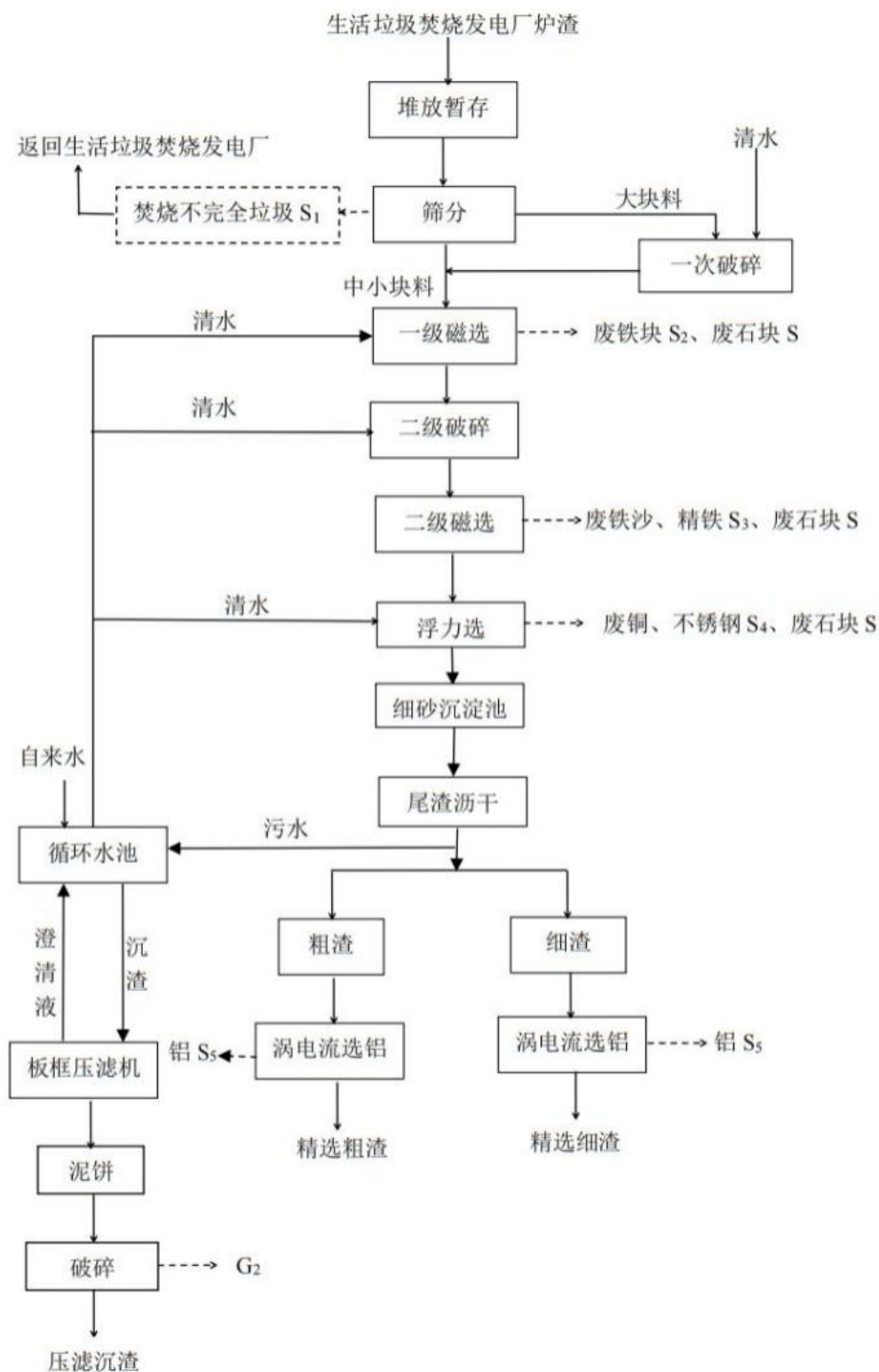
图 2-4 现有炉渣分选生产线产排污节点图
