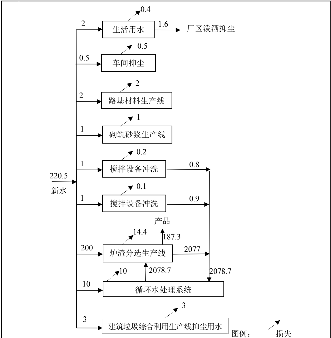
图 2-2 项目建成后全厂给排水平衡图（单位：m³/d）
