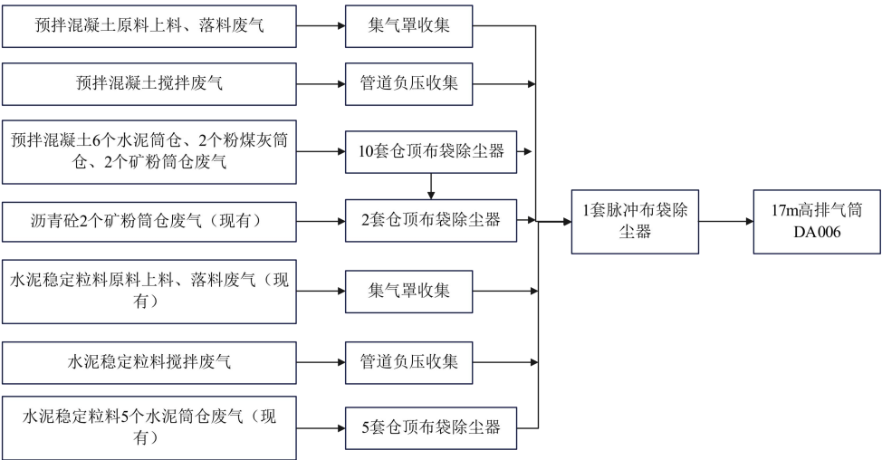
图 4-1 废气收集及环保设施示意图
