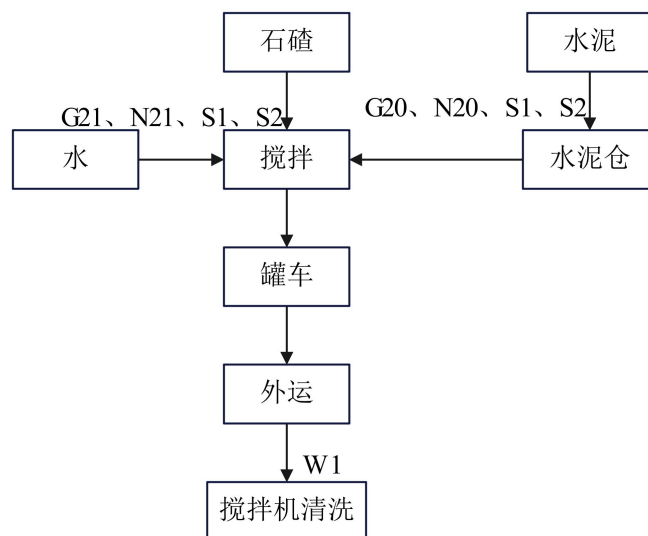
图 2-8 沥青砼生产工艺流程及排污节点图
