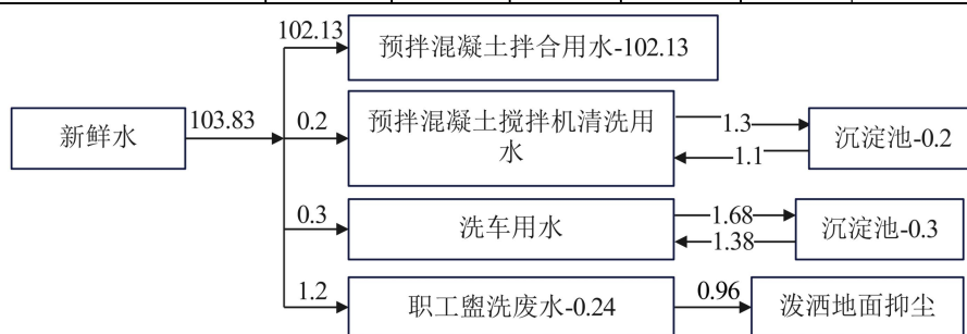
图 2-1 本项目给排水平衡图 \text{m}^3/\text{d}
