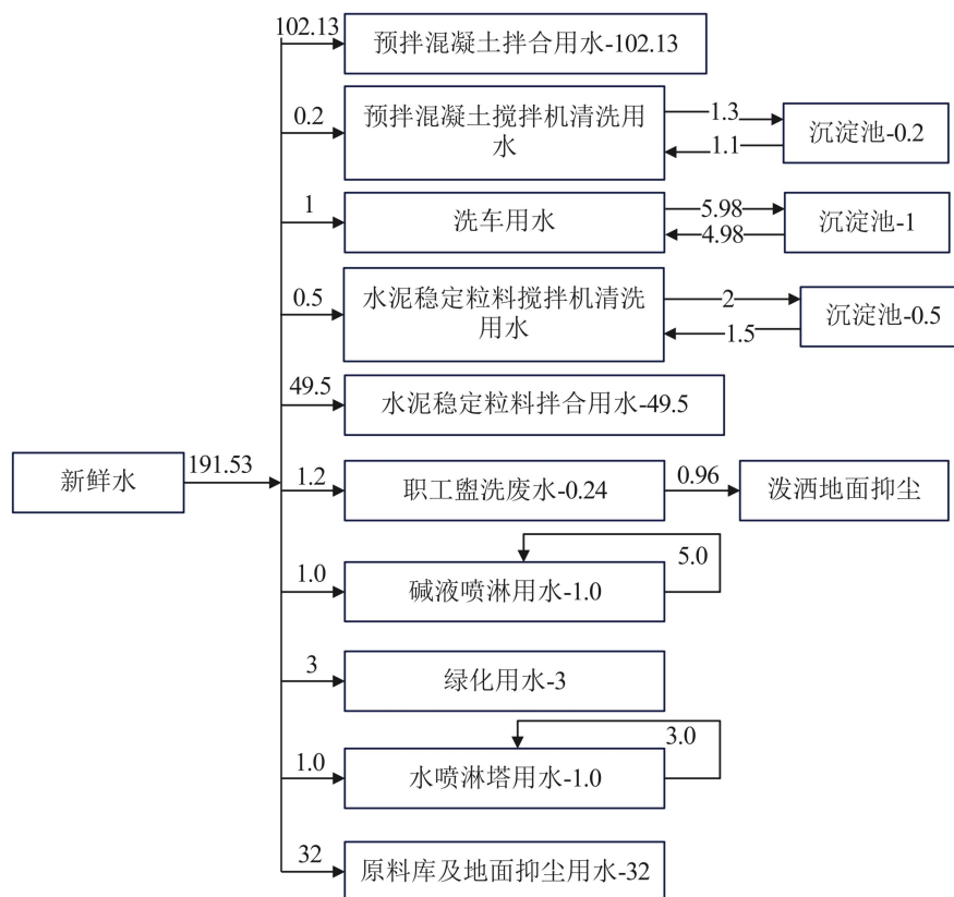
图 2-2 扩建后全厂给排水平衡图 m³/d
